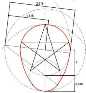
Vergleich mit Zeichnungen aus einer Patentschrift von V. Schauberger zur Gestaltung von Rohren:
